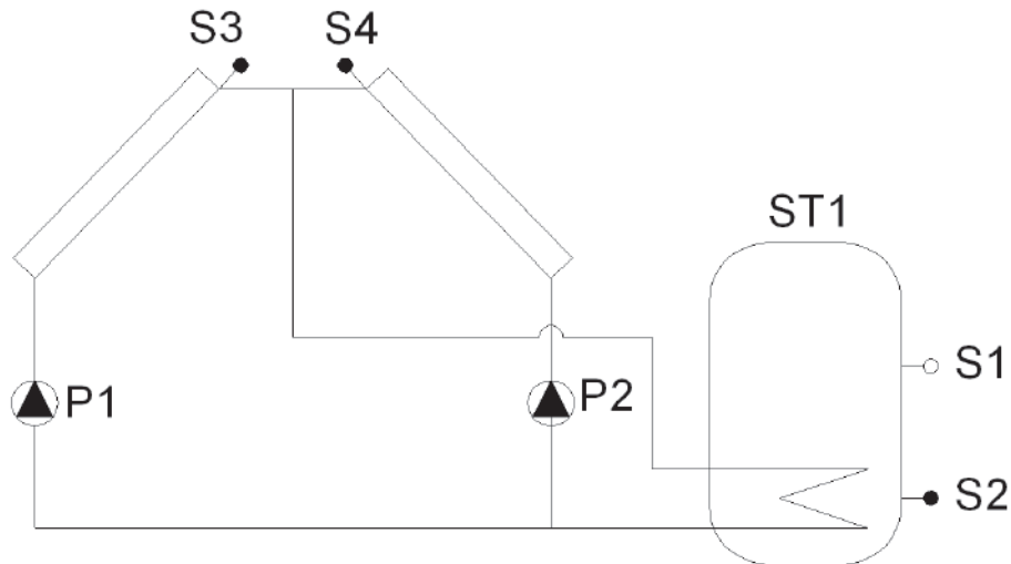
Schema 4 - sistema est / ovest con due pompe
