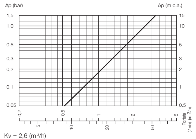
Caratteristiche idrauliche
